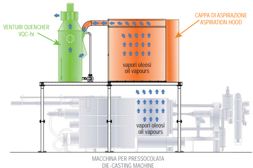
Nuovo Venturi-Quencher abbattimento vapori oleosi da singola macchina di pressocolata New Venturi-Quencher oil vapours treatment from single die-casting machine
